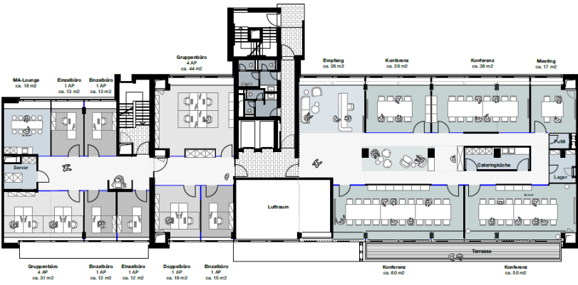
1. Obergeschoss | Musterplanung | Konferenz
